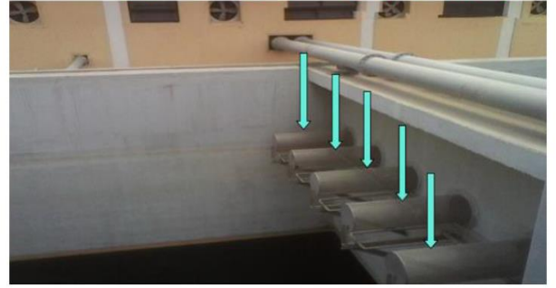
مناخل خروج المياه من حوض ال MBBR لمنع هروب الحاملات البلاستيكية.
